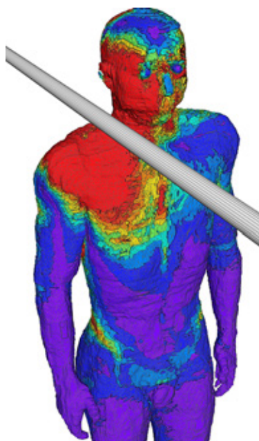
Figura D14 — Esempio 2: Distribuzione del campo elettrico indotto derivante dall'esposizione a un cavo a 50 Hz collocato vicino alla testa
