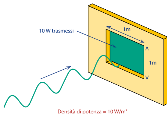
Figura C4 — La densità di potenza è la potenza irradiata per ciascuna unità di area
