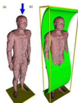
Figura D11 — Esempio 1: Modello umano esposto a un campo elettromagnetico riflesso nella zona occupata dall'essere umano. Questa regione è indicata con un riquadro giallo. L'onda stazionaria è indicata in verde
