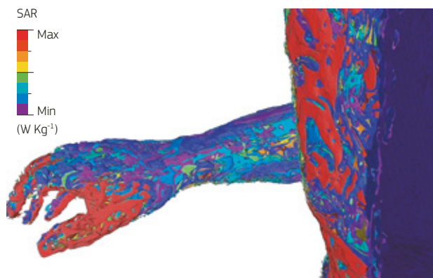
Figura D10 — Determinazione delle grandezze dosimetriche, in questo caso il SAR nella mano e nel tronco derivante dall'esposizione a un cavo non schermato, per la comparazione diretta con i VLE. La direttiva raccomanda questo approccio per dimostrare la conformità nel caso di sorgenti di campo elettromagnetico molto localizzate situate a pochi centimetri dal corpo
