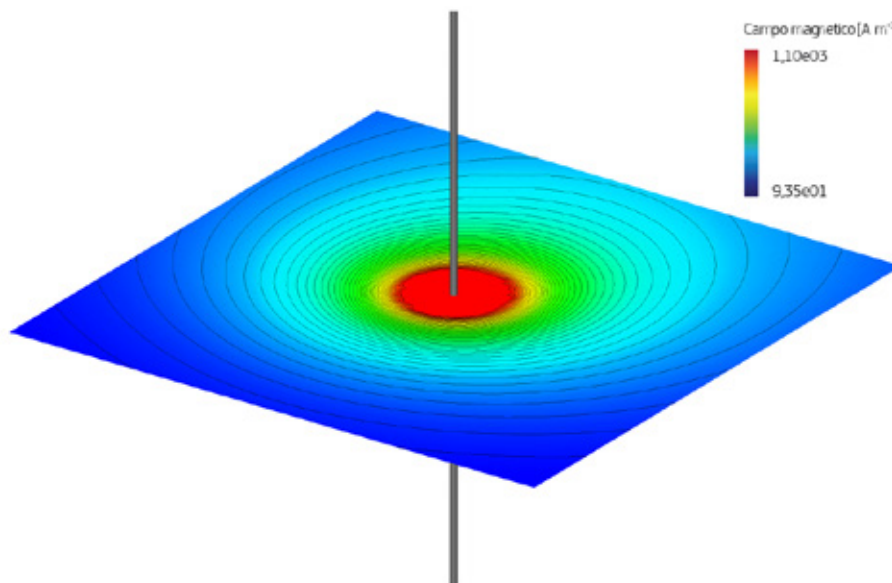
Figura C3 — La distribuzione spaziale dell'intensità di campo magnetica intorno a un cavo da 50 Hz che conduce una corrente di 70 A
